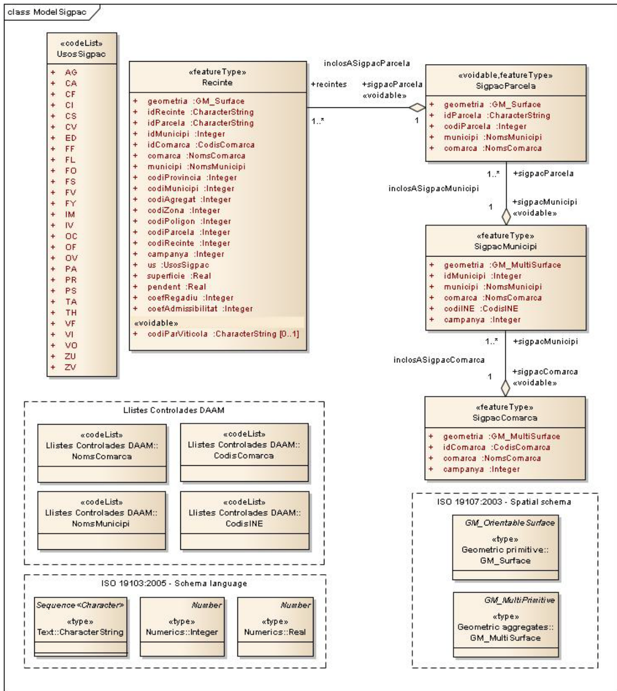
Figura 1 - Diagrama de classes UML del model de dades del SIGPAC v1.1
